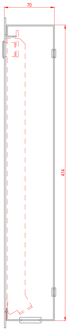
Zijaanzicht
